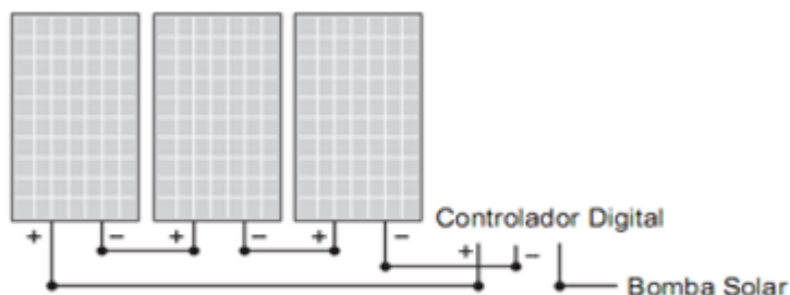
3 paneles solares de 550 W
